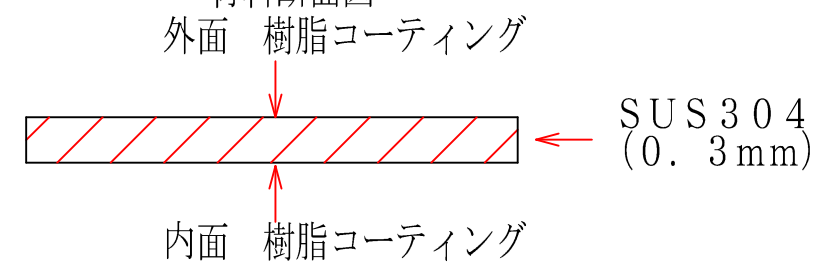
材料断面図
